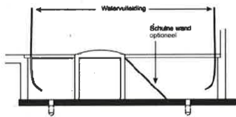
Doorsnede variant bolle vloer
