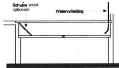
Doorsnede A-A (variant)
