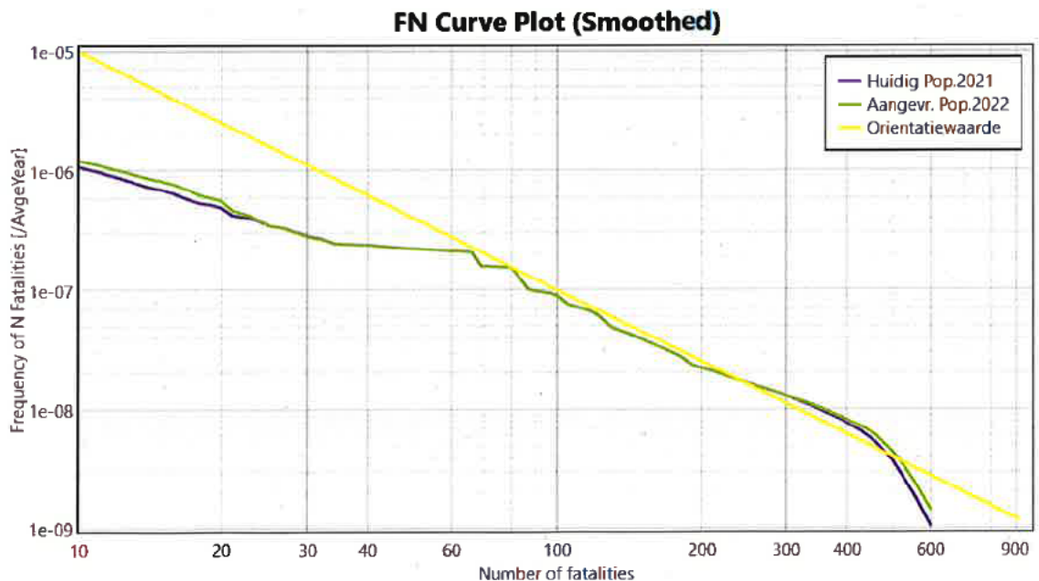
Figuur 2: Groepsrisico
