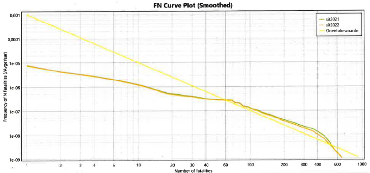
Figuur 2 Groepsrisico
